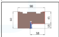
OŚCIEŻNICA FD-25/12: SENATOR E, HETMAN 55, BATORY 55, MOZART, AMADEO, VERDI OŚCIEŻNICA STALOWO-DREWNIANA: SENATOR E
