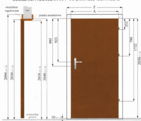
OŚCIEŻNICA REGULOWANA
