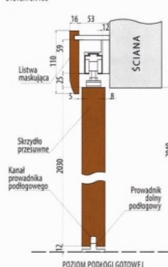
POZIOM PODŁOGI GOTOWEJ
