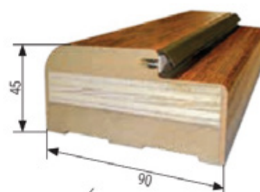
Ościeżnica stała wzmocniona OW-01
