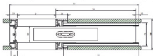
WYMIARY SYSTEMU PODWÓJNEGO (PODANE WYMIARY W MM)
