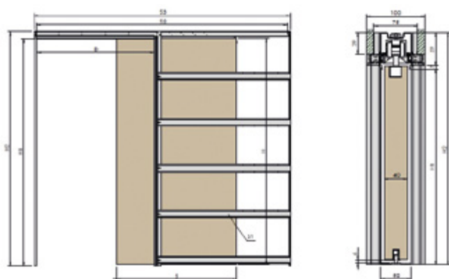
WYMIARY SYSTEMU POJEDYŃCZEGO (PODANE WYMIARY W MM)
