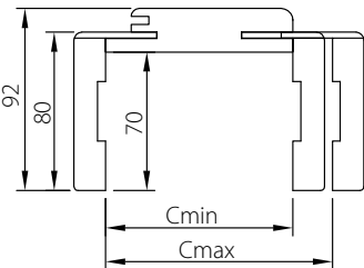
Przekrój OR z kątownikiem 80
