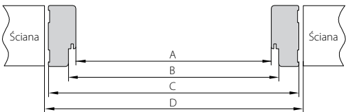
Przekrój poziomy
