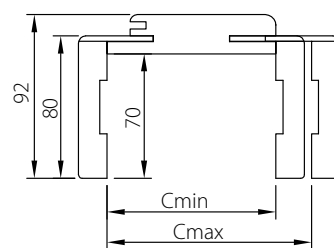
Przekrój OR z kątownikiem 80
