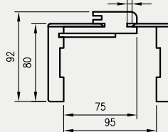
Przekrój ORB 095-300
