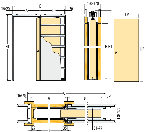
System przesuwny wewnętrzny pojedynczy
