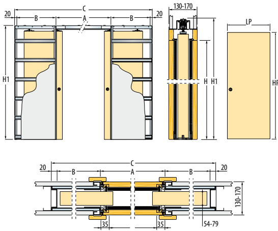
System przesuwny wewnętrzny podwójny
